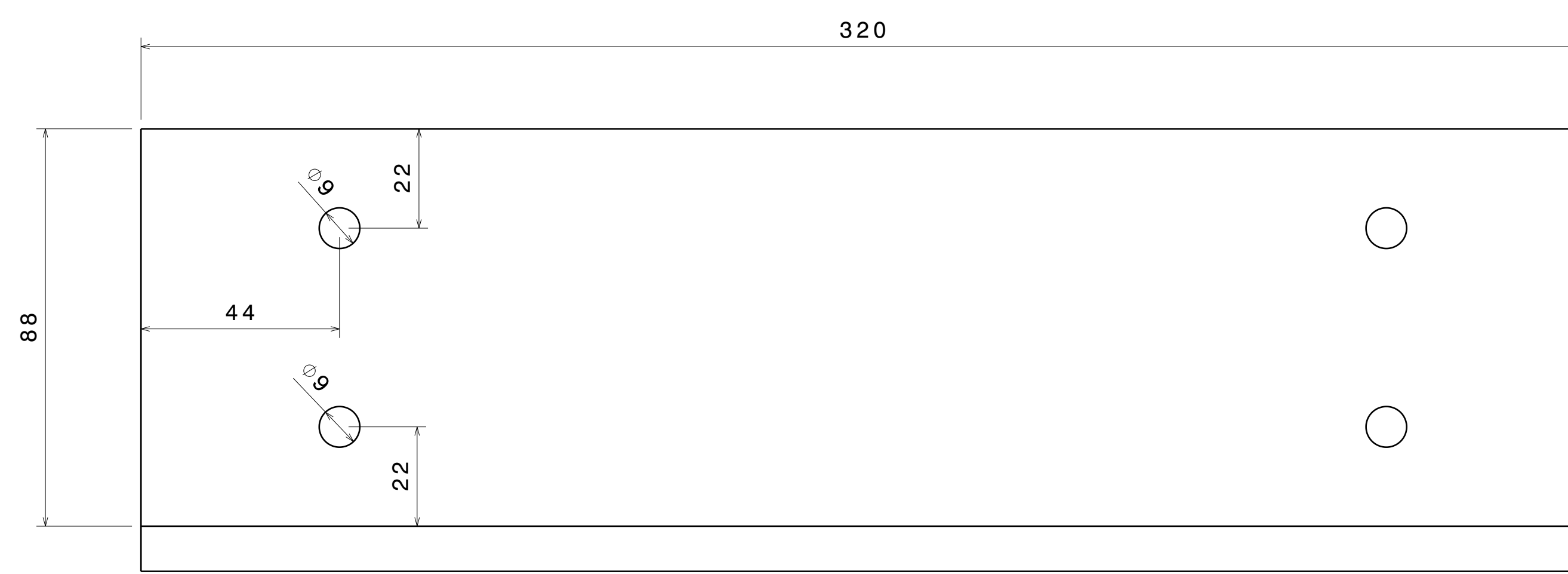
Vorderansicht Maßstab: 1:1
