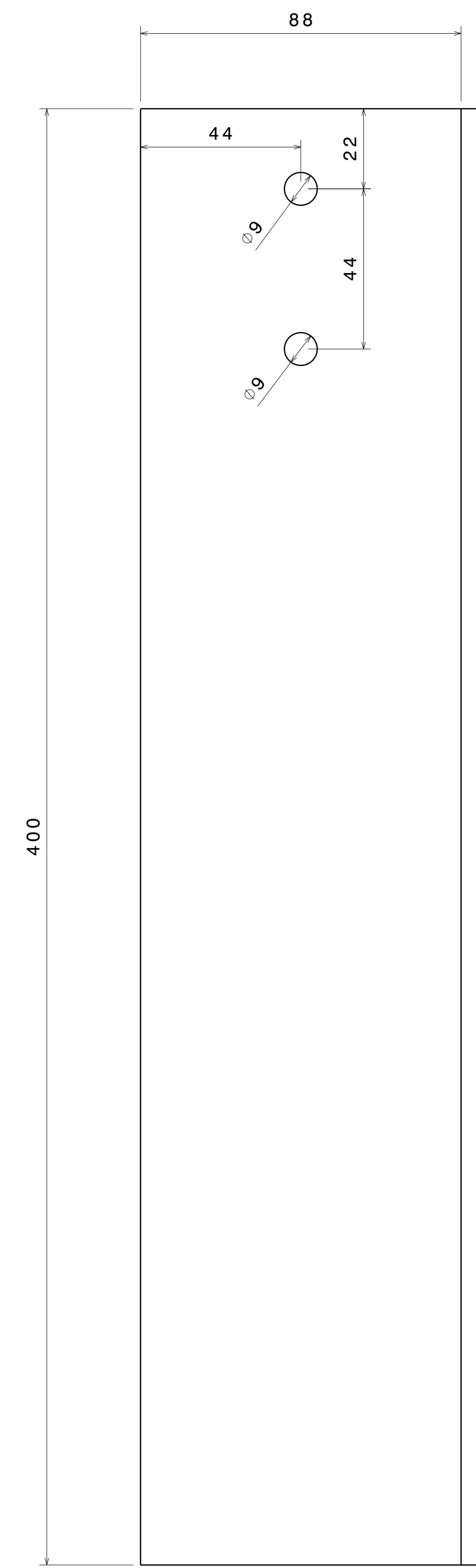
Vorderansicht Maßstab: 1:1
